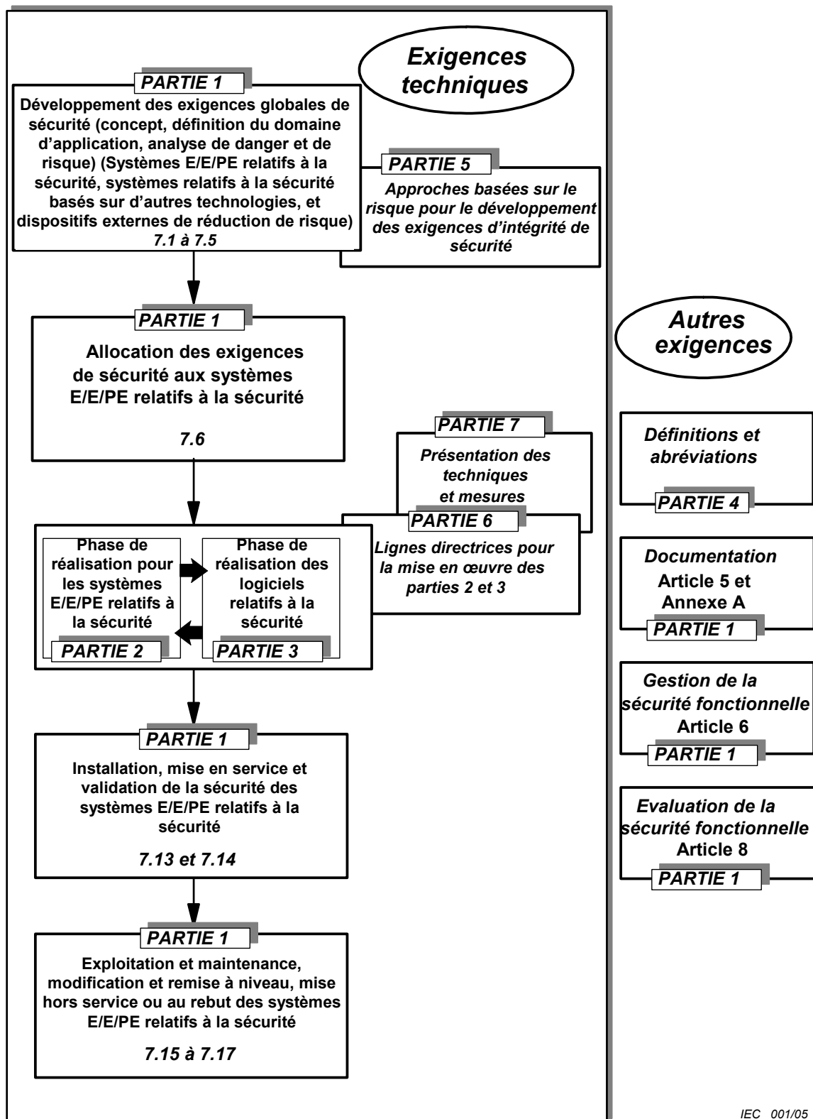
Figure 1 – Carte des exigences pour les parties 1 à 7 de la CEI 61508
